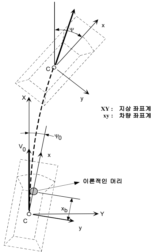
그림 2.5 차량과 지상좌표
