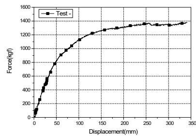
정적시험 결과(예)
