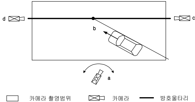
그림 3.1 방호울타리 및 전이구간 충돌시험 카메라 배치도
