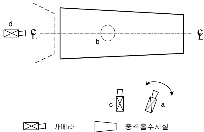
그림 3.2 충격흡수시설 및 단부처리시설 충돌시험 카메라 배치도
